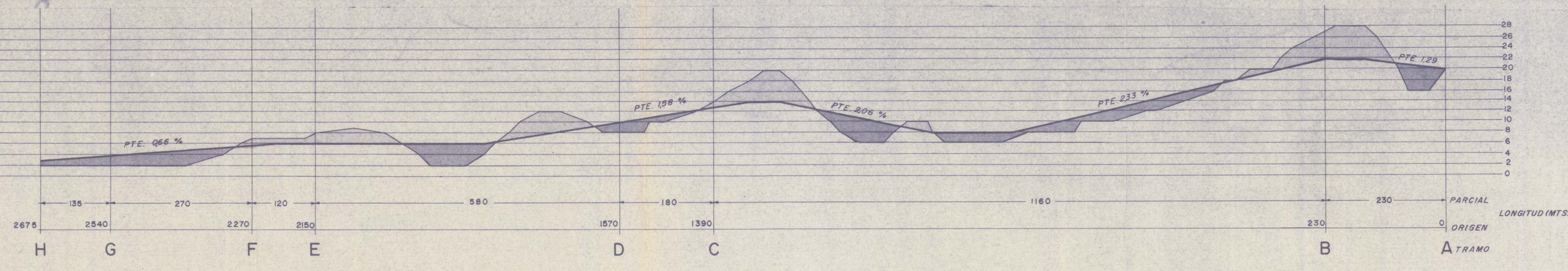
PERFIL LONGITUDINAL
